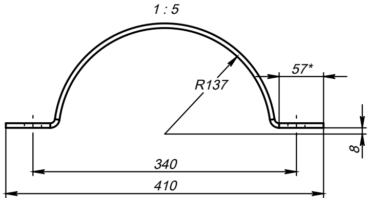
Поз.10 (Полухомут)
