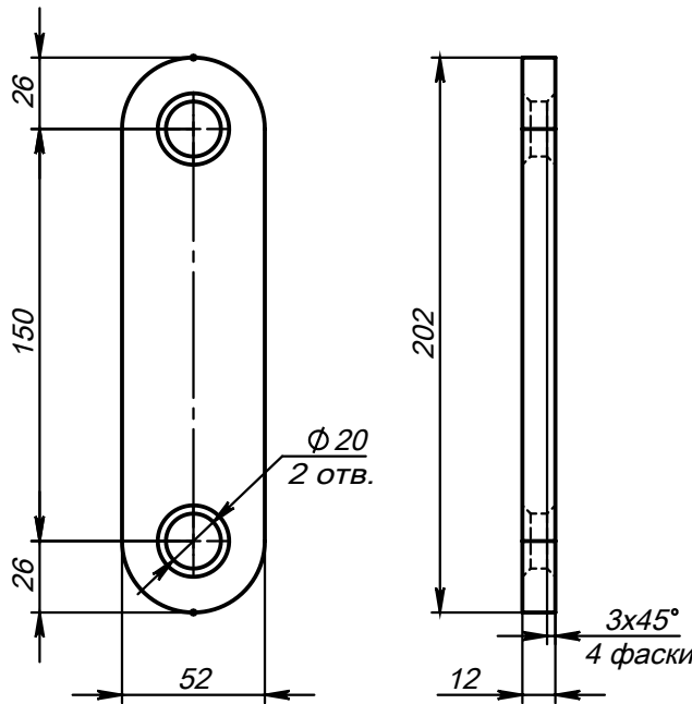
Поз.9 (Серьга)
