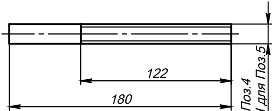
Поз.4 и Поз.5 (Шпилька)
