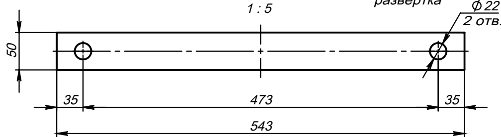
Поз.10 (Полухомут) развёртка
